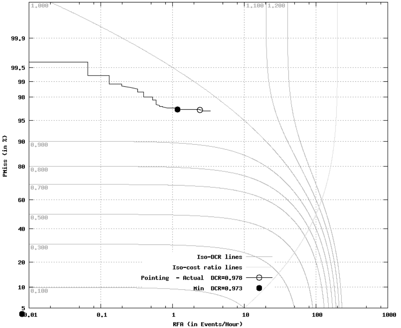
DET for BJTU-SED_1 : BJTU-SED_2011_retroED_EVAL11_ENG_s-camera_p-SYS_1
