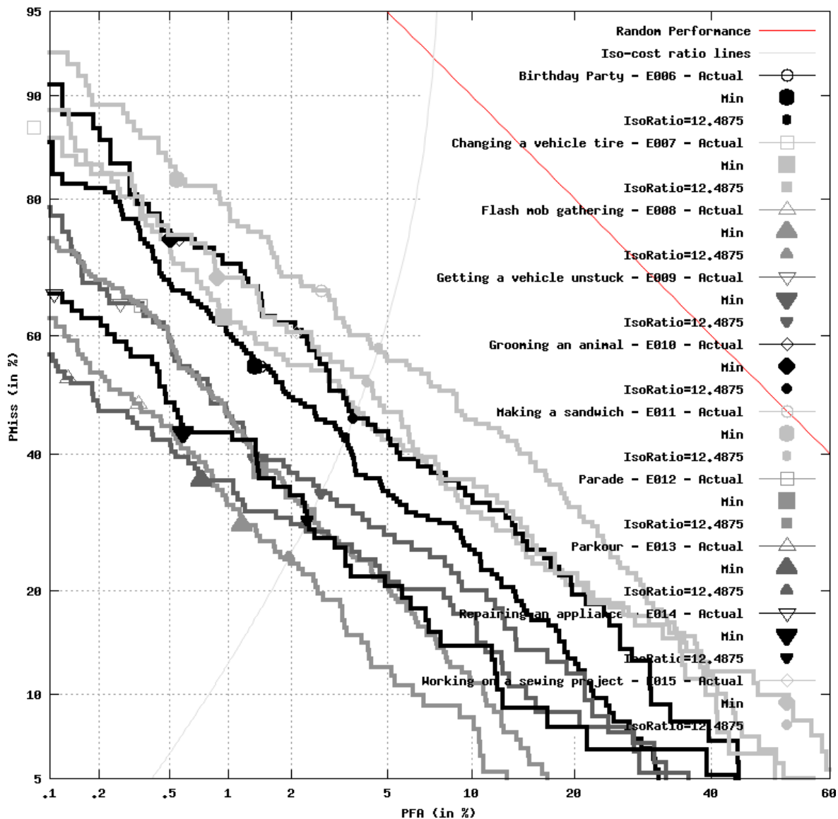
DET for INRIA-LEAR_4 : INRIA-LEAR_MED11_MED11TEST_MEDFull_AutoEAG_p-mbh_1
