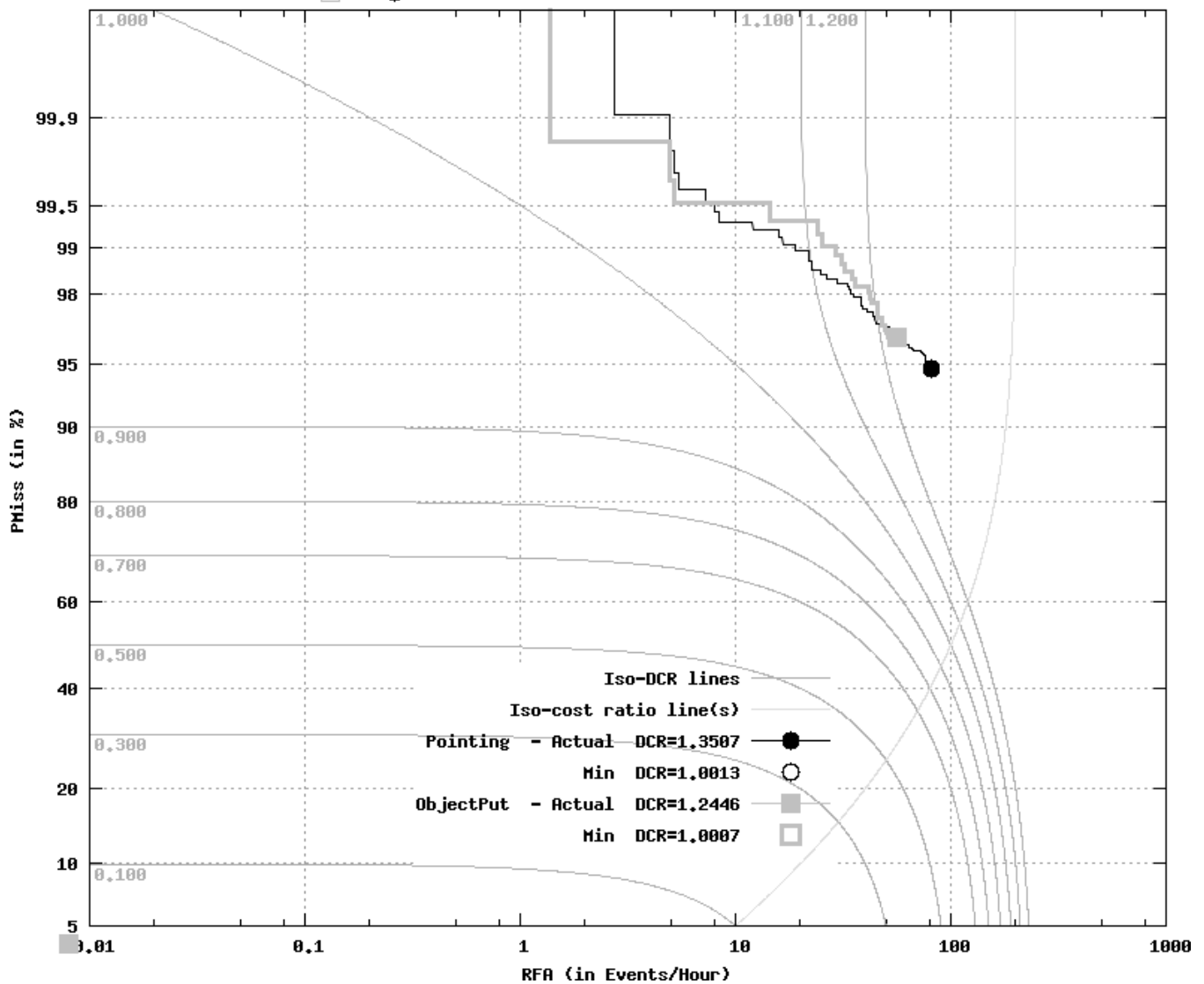
DET for SED12_dcu-savasa_retroED_EVAL12_3 : dcu-savasa_2012_retroED_EVAL12_ENG_s-camera_c-uuid_1
